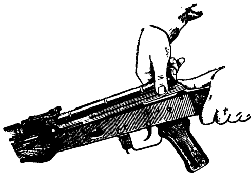
Рис. 5. Отделение крышки ствольной коробки
