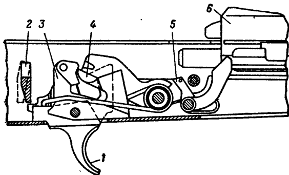
Рис. 44. Положение частей ударно-спускового механизма перед выстрелом:
