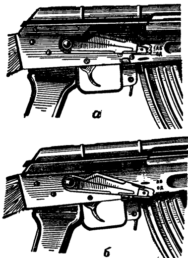
Рис. 58. Установка переводчика на необходимый вид огня: а — для ведения автоматического огня; б — для ведения одиночного огня
