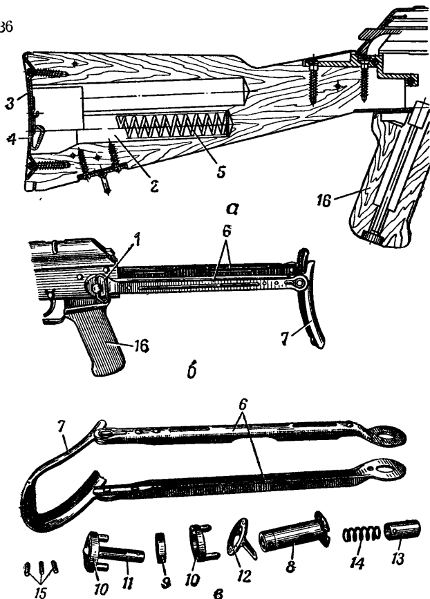
Рис. 30. Приклад и пистолетная рукоятка: а — деревянный приклад; б — складывающийся приклад; в — складывающийся приклад в разобранном виде; 1 — антабка для ремня; 2 — гнездо для принадлежности; 3 — затылник; 4 — крышка; 5 — пружина для выталкивания пеныла с принадлежностью; 6 — тяги; 7 — плечевой упор; 8 — соединительная втулка; 9 — гайка; 10 — фиксаторы приклада; 11 — соединительный стержень; 12 — шайба с антабкой; 13 — колачок; 14 — пружина; 15 — шпильки; 16 — пистолетная рукоятка
