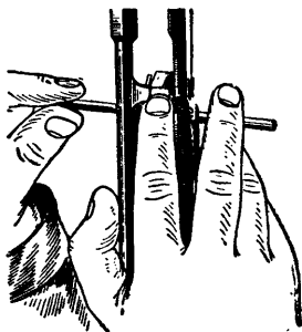
Рис. 20. Вставление оси автоспуска
