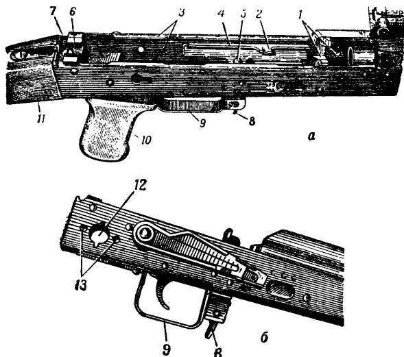
Рис. 27. Ствольная коробка:
