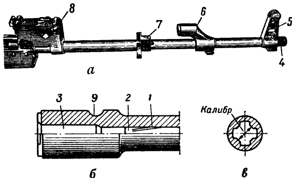
Рис. 25. Ствол:
