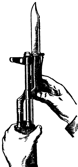
Рис. 24. Отмыкание штыка-ножа
