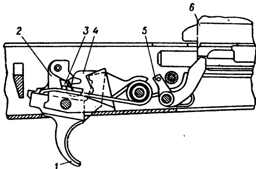
Рис. 45. Положение частей ударно-спускового механизма после выстрела при переводчике, установленном на одиночный огонь:
