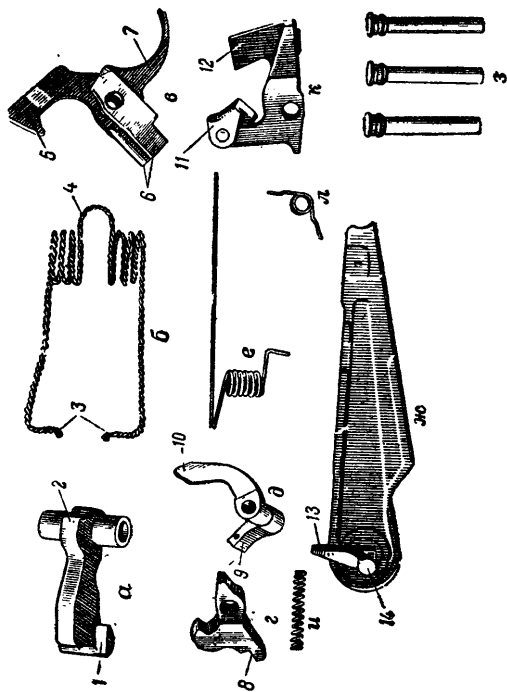
Рис. 35. Части ударно-спускового механизма:
