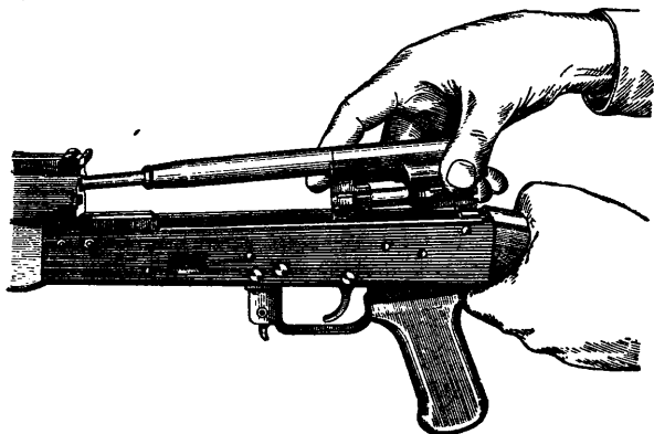
Рис. 7. Отделение затворной рамы с затвором
