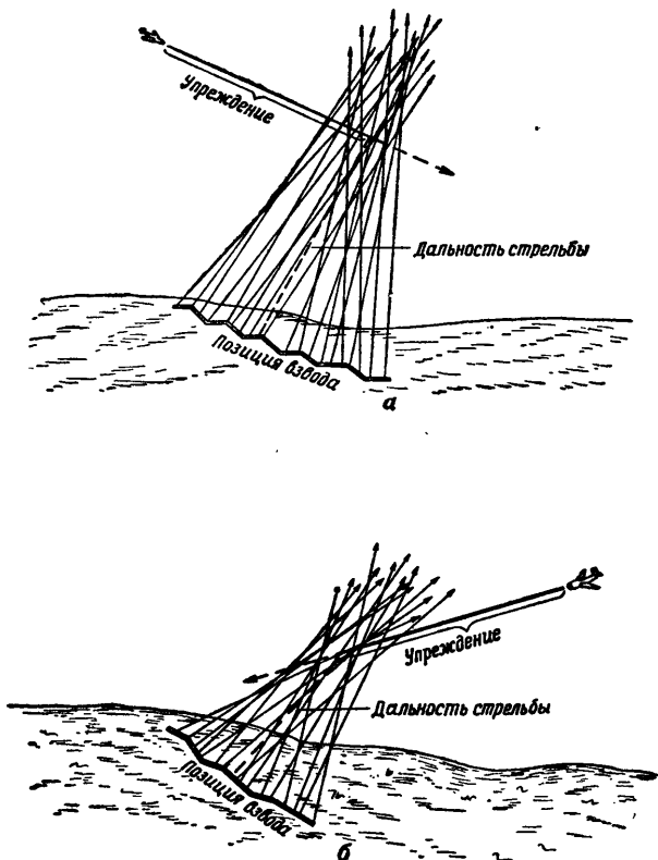
Рис. 84. Ведение огня заградительным способом по самолету:
