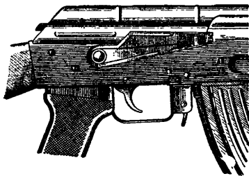
Рис. 53. Автомат поставлен на предохранитель
