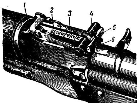
Рис. 28. Прицел:
