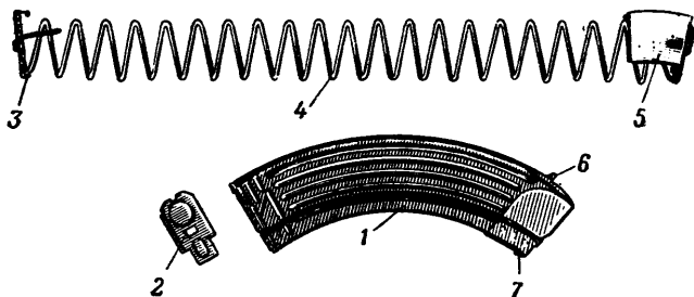
Рис. 37. Магазин:
