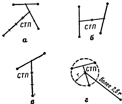
Рис. 47. Определение средней точки попадания:
