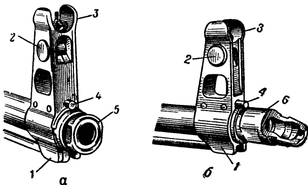
Рис. 26. Основание мушки:
