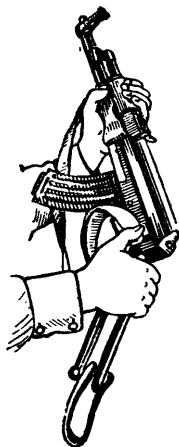
Рис. 66. Складывание приклада
