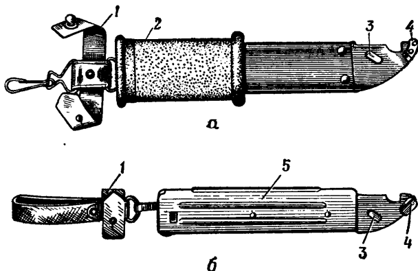
Рис. 39. Ножны:
