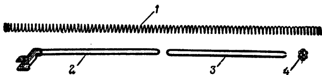
Рис. 33. Возвратный механизм:
