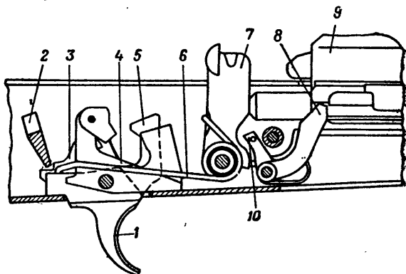
Рис. 43. Положение частей ударно-спускового механизма до заряжания при включенном предохранителе и спущенном курке:
