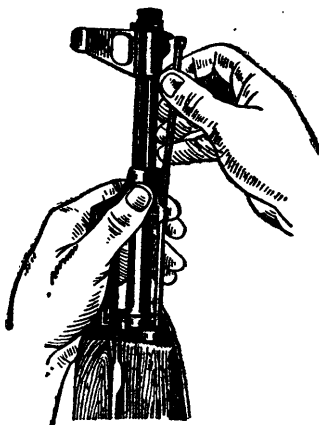
Рис. 4. Отделение шомпола
