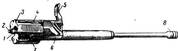
Рис. 31. Затворная рама с газовым поршнем:
