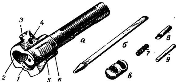
Рис. 32. Затвор:
